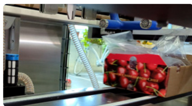
5 Sortie des boîtes
